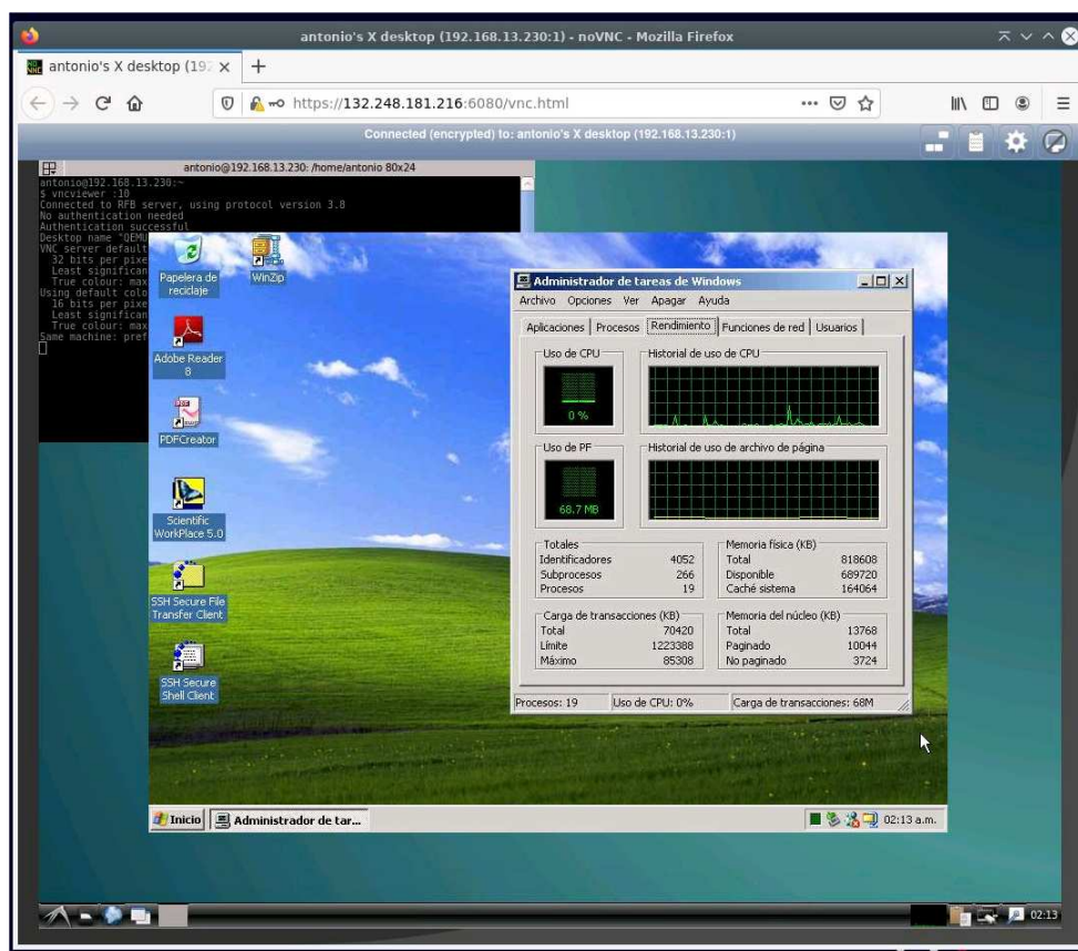
Figura 21: Uso de noVNC desde el navegador Mozilla Firefox sobre un equipo en red que soporta ejecución de máquinas virtuales sobre Debian GNU/Linux.
