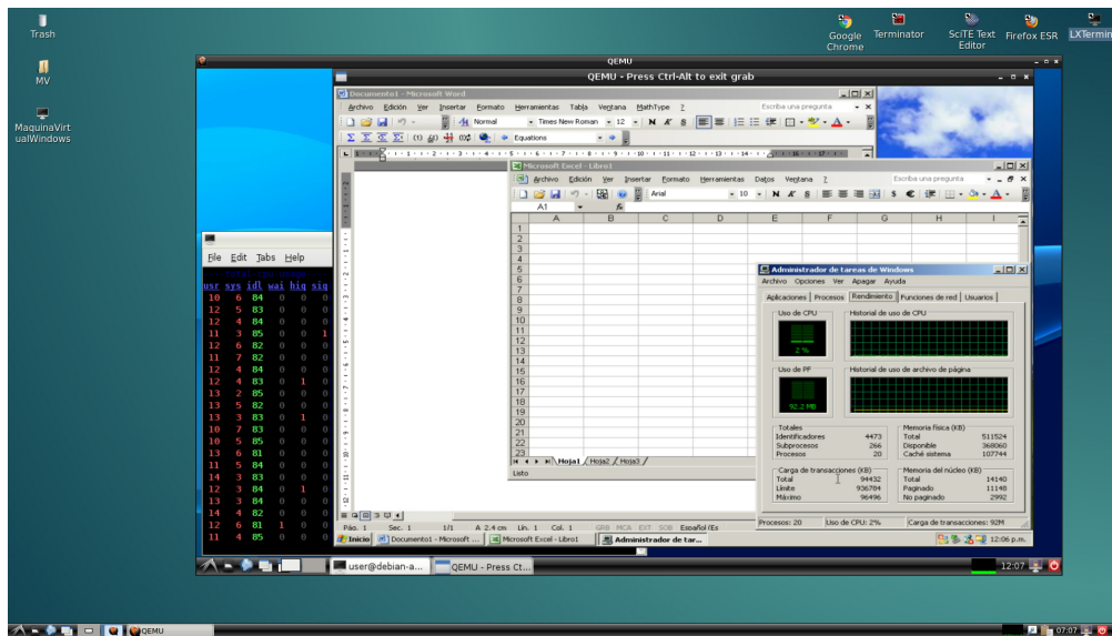
Figura 20: Sobre un equipo AMD de gama baja y 4 GB de RAM, se muestra el uso de una virtualización sobre otra virtualización y corriendo dentro de ella, una máquina virtual con Windows XP en la cual se muestra el uso de RAM y CPU dentro de la misma.
