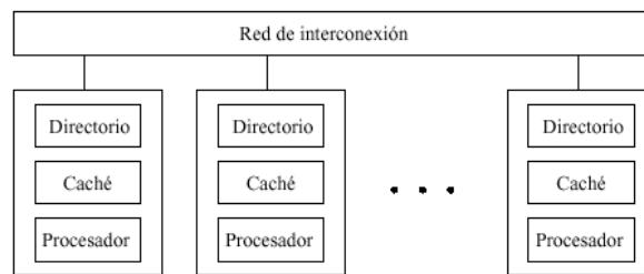
Figura 12: Ejemplo de COMA
