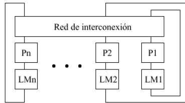
Figura 11: Acceso no uniforme a la memoria NUMA
