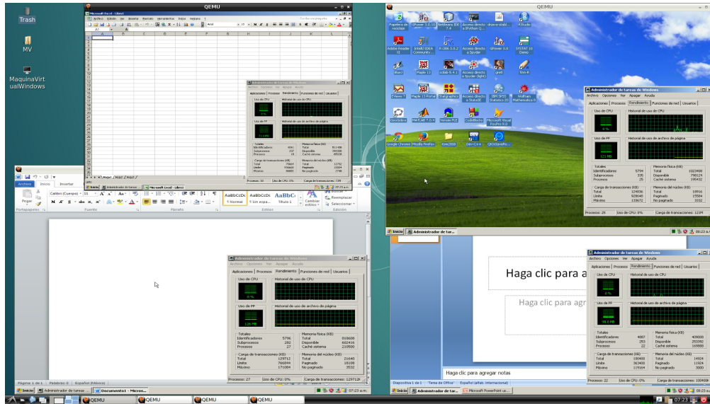
Figura 17: Sobre un equipo AMD de gama baja y 4 GB de RAM, usando como sistema operativo huésped un Linux Debian estable, se ejecutan 4 máquinas virtuales (mediante KVM) de Windows XP con diferentes aplicaciones y dentro de cada una de ellas se muestra la RAM asignada, la usada en ese momento, el uso de CPU de cada máquina virtual, entre otros datos.
