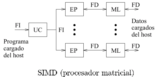
Figura 6: Ejemplo de máquina SIMD
