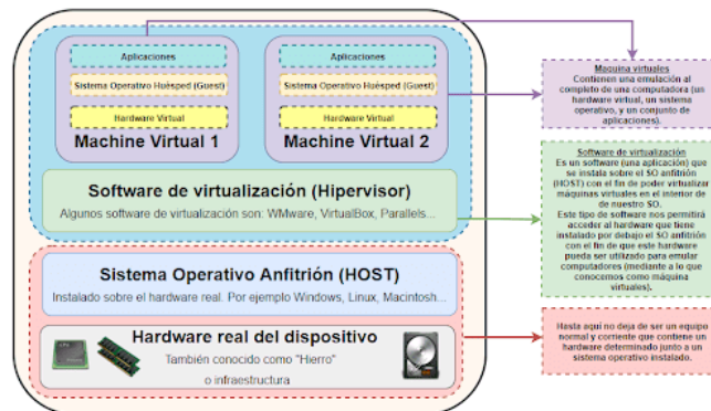
Figura 18: Qué es una Máquina Virtual
