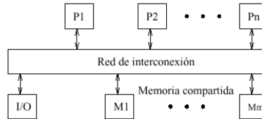
Figura 10: Acceso Uniforme a la memoria UMA
